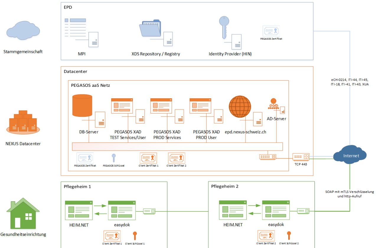
Abbildung: Systemarchitektur mit NEXUS / PEGASOS als EPD-Enabler/Archiv
